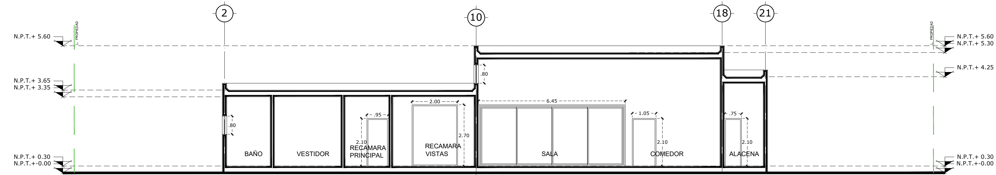
SECCION B-B TRANSVERSAL ESTADO ACTUAL ESCALA 1 : 100
