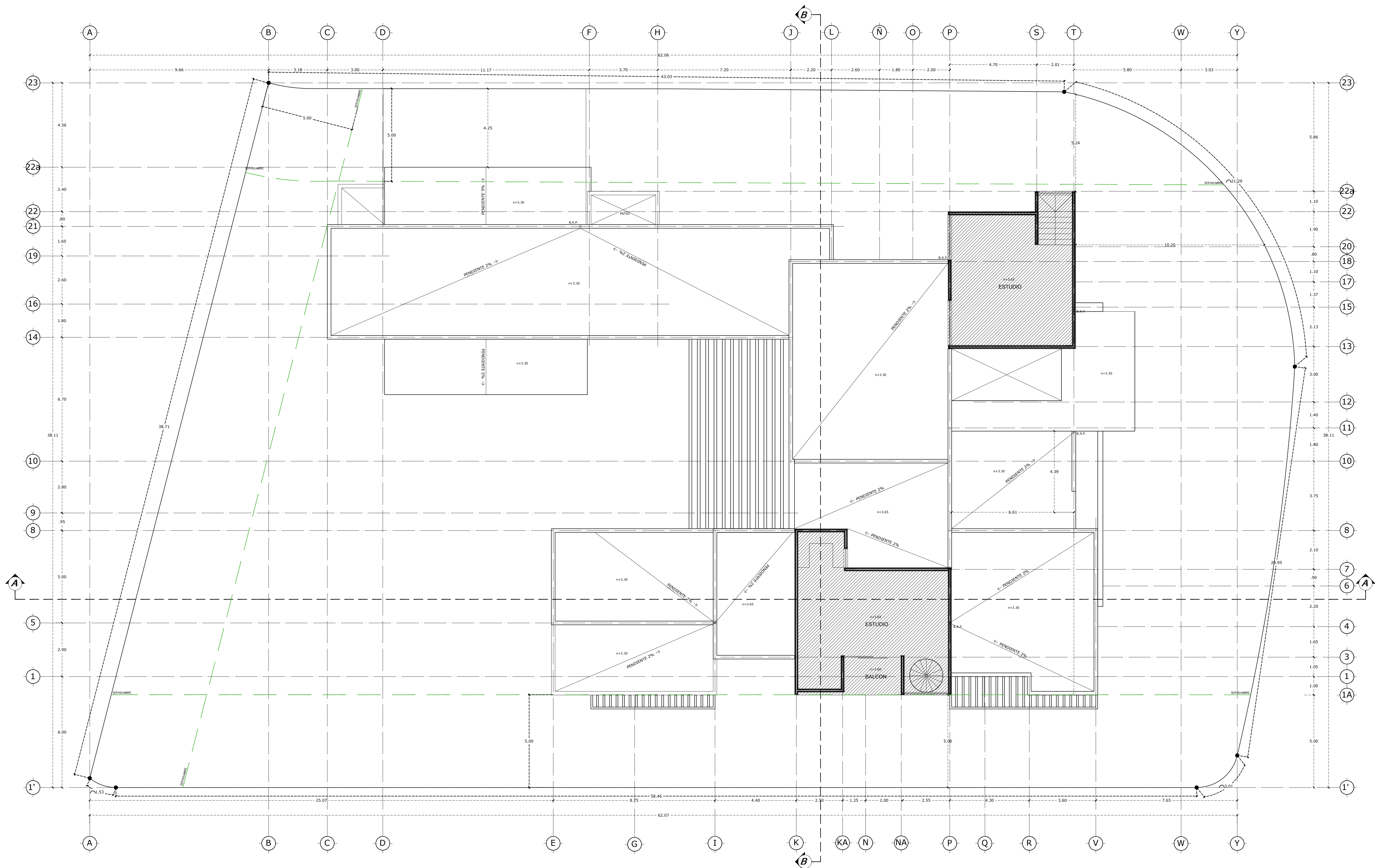
PLANTA ALTA ESTADO PROPUESTO ARQUITECTONICA ESCALA 1:100
