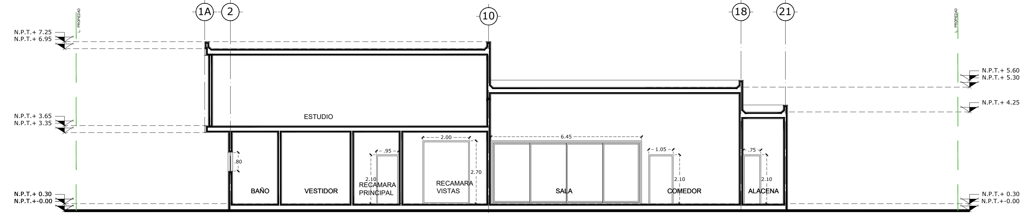
SECCION B-B TRANSVERSAL ESTADO PROPUESTO ESCALA 1 : 100
