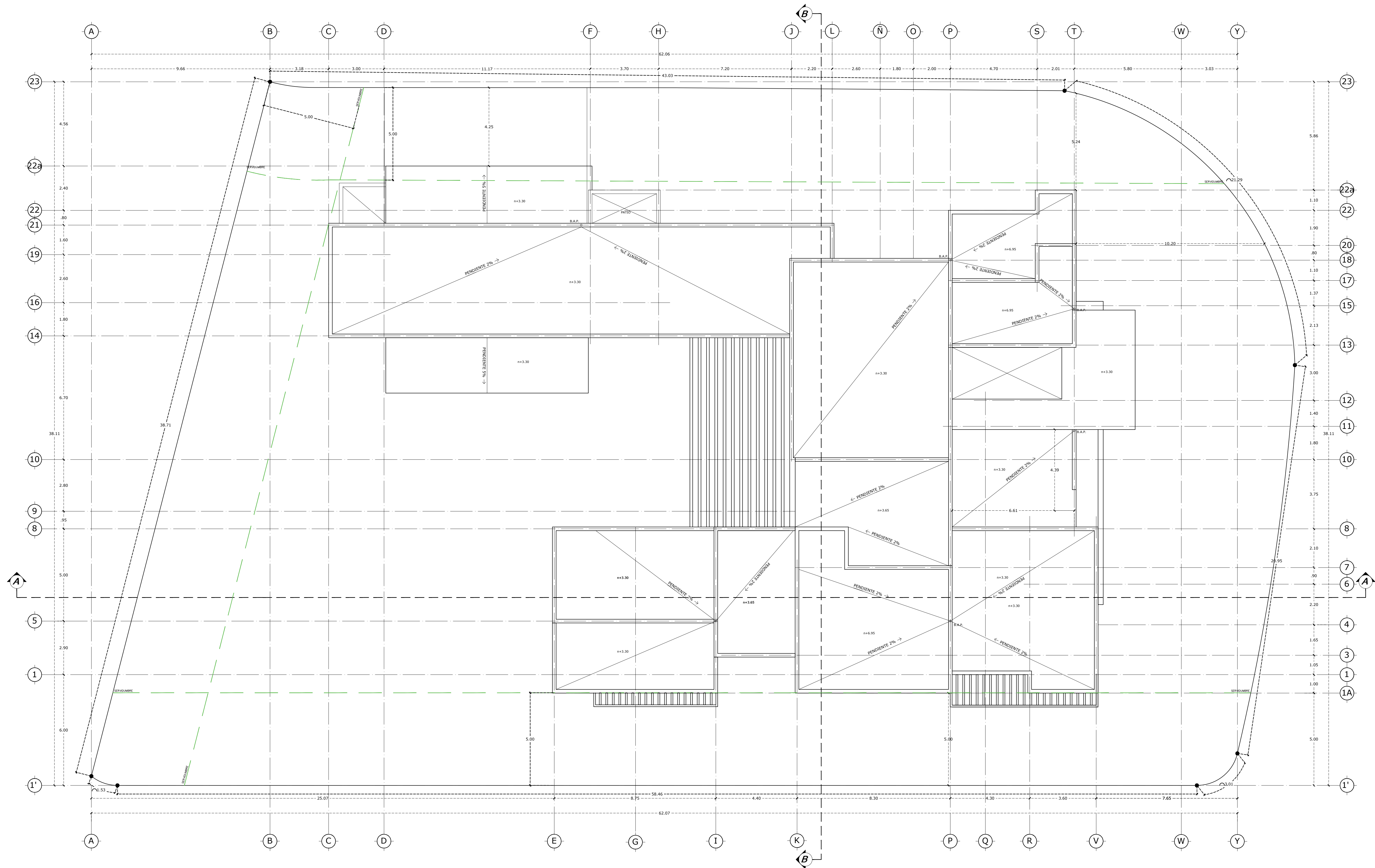
PLANTA DE AZOTEA ESTADO PROPUESTO ARQUITECTÓNICA ESCALA 1:100
