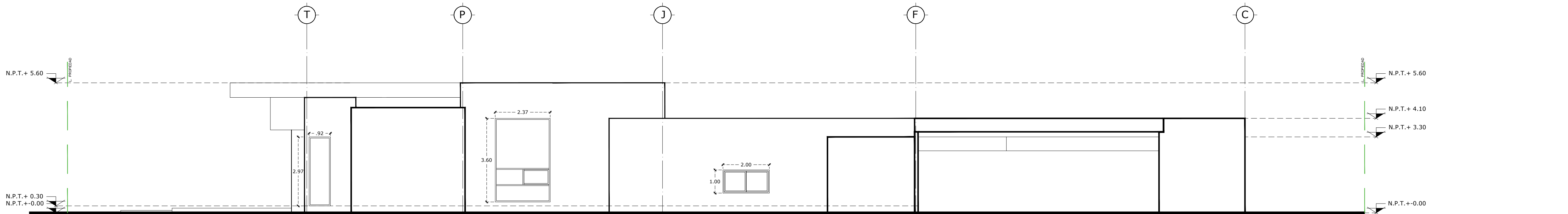
ALZADO ESTADO ACTUAL 04
